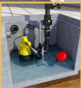
AG10 - Alarmtoestel met kogeldompelschakelaar voor pompenschachten
